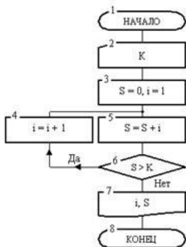
Рис. 19. Разветвляющийся алгоритм
