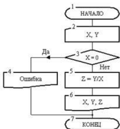
Рис. 18. Разветвляющийся алгоритм
